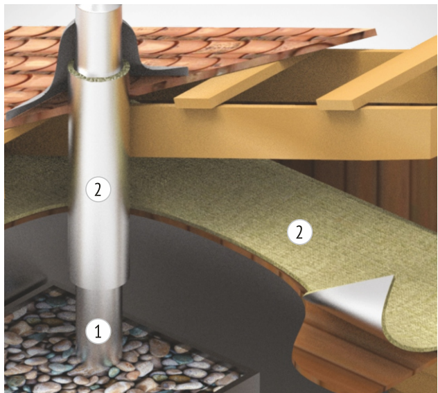
1. Дымоход 2. МБОР
