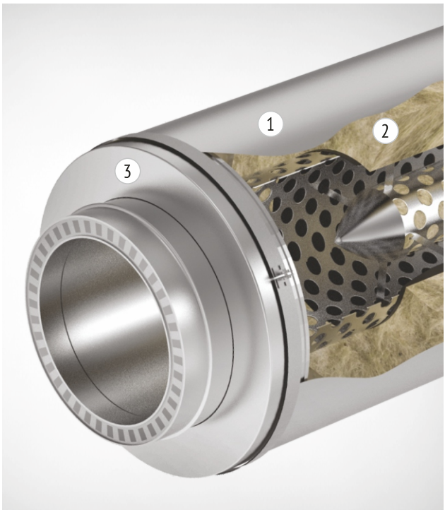
1. Защитный кожух 2. БСТВ 3. Глушитель
