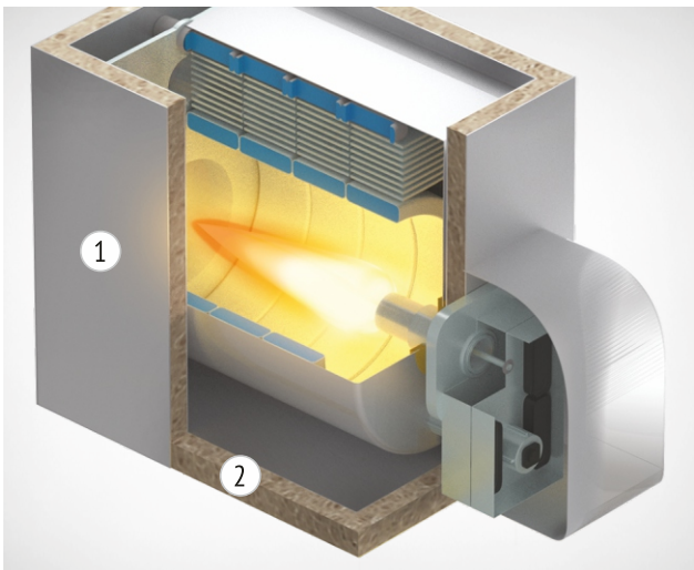
1. Кожух 2. БВТМ-ПМ/БВТМ-К
