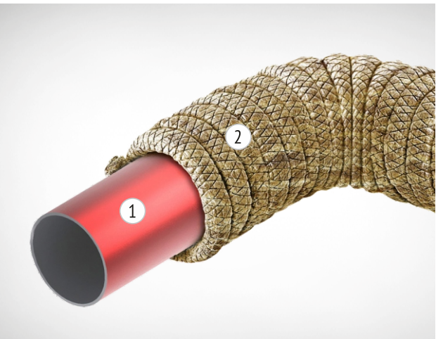
1. Трубопровод 2. Шнур базальтовый теплоизоляционный «ШБТизол»
