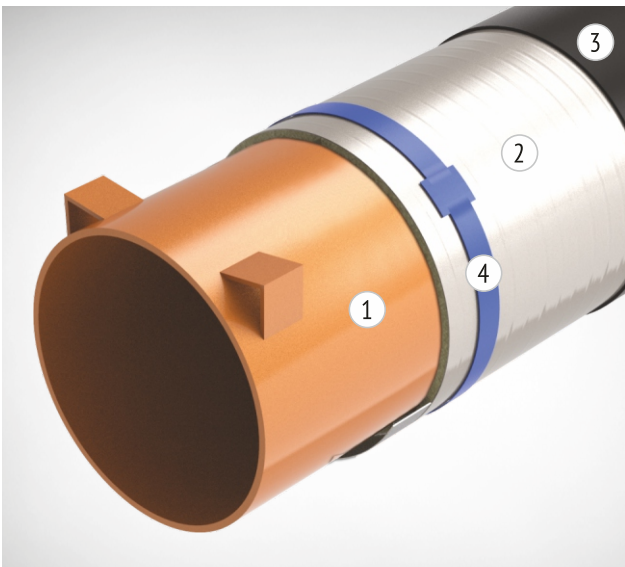
1. Трубопровод 2. МБОР 3. Защитное покрытие 4. Бандаж
