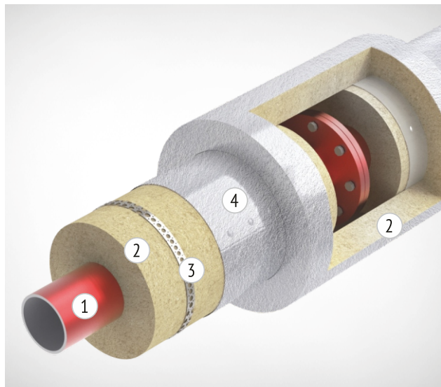
1. Труба 2. Цилиндры EURO-ШЕЛЛ 3. Бандаж с пряжкой 4. Защитное покрытие
