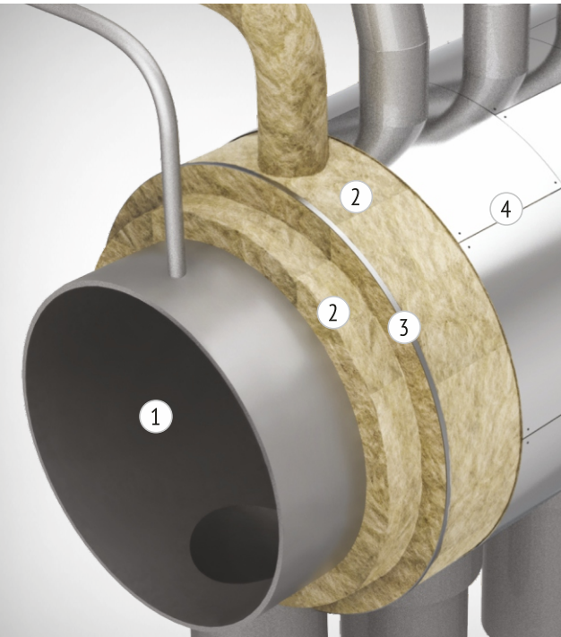
1. Оборудование 2. МПБ 3. Опорная конструкция кожуха 4. Защитный кожух
