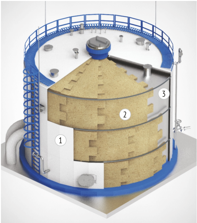
1. Защитный кожух 2. МПБ 3. Корпус
