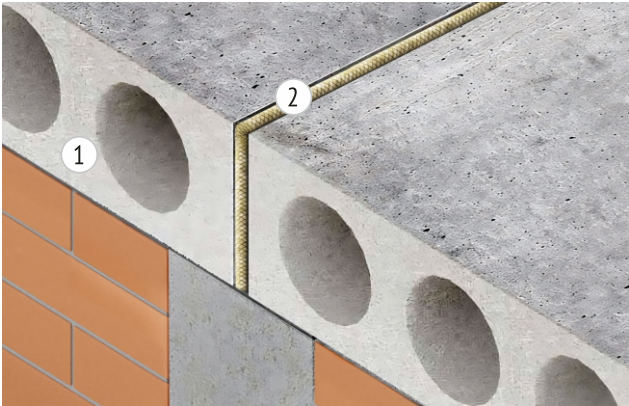
1. Железобетонная плита 2. Шнур базальтовый теплоизоляционный «ШБТизол»
