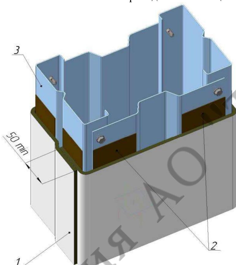
Рисунок В1. Схема огнезащиты конструкции замкнутого профиля
