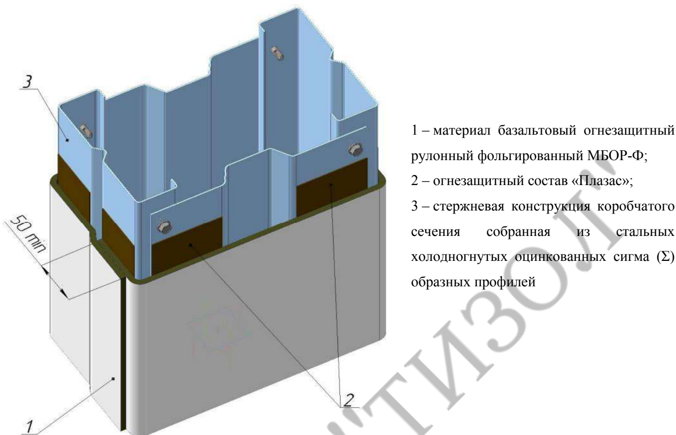
Рисунок 2. Схема огнезащиты конструкции замкнутого профиля
