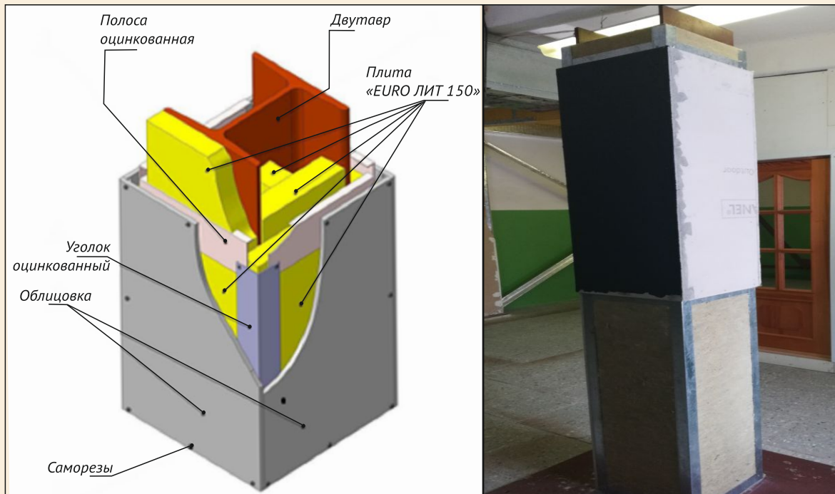
Схема монтажа системы «ЕТ Металл плюс»
