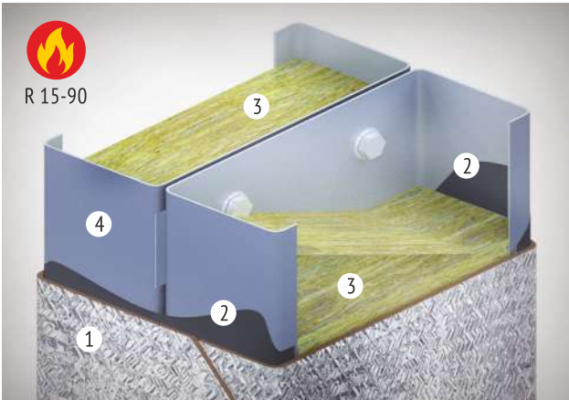
Огнезащита конструкций из профилей, собранных двутавром 1. Материал рулонный МБОР-Ф 2. Огнезащитный состав «ПЛАЗАС» 3. Огнезащитная плита «EURO-ЛИТ» 4. Холодногнутой оцинкованный профиль ЛСТК
