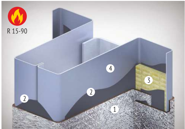
Огнезащита конструкций из профилей Z 1. Материал рулонный МБОР-Ф 2. Огнезащитный состав «ПЛАЗАС» 3. Огнезащитная плита «EURO-ЛИТ» 4. Холодногнутой оцинкованный профиль ЛСТК
